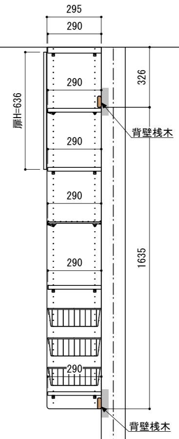
A-A' 断面
