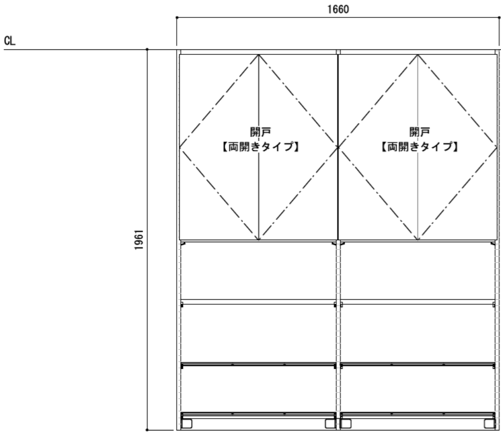
正面図（外観）
