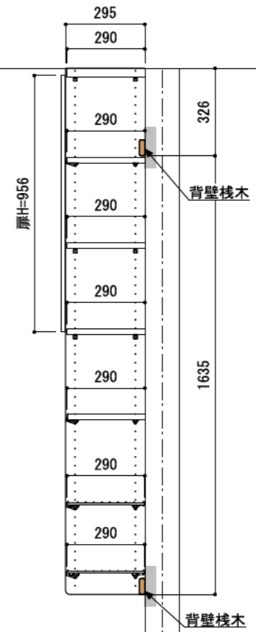
A-A' 断面
