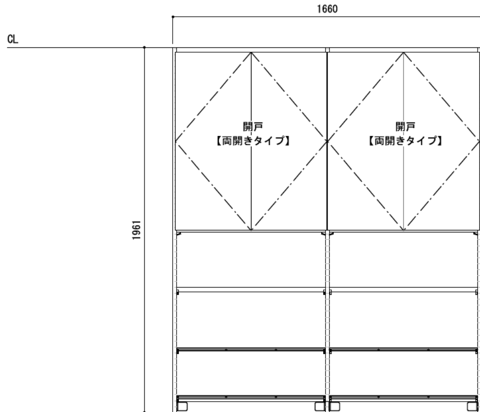
正面図（外観）
