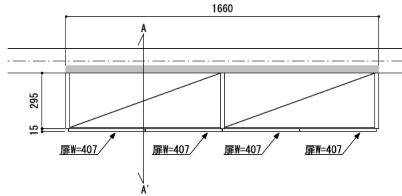
正面図（外観）
