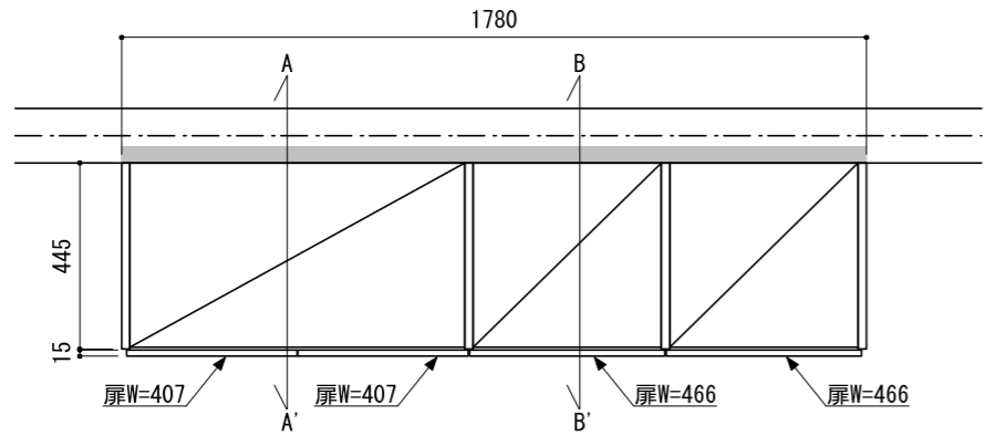
正面図（外観）
