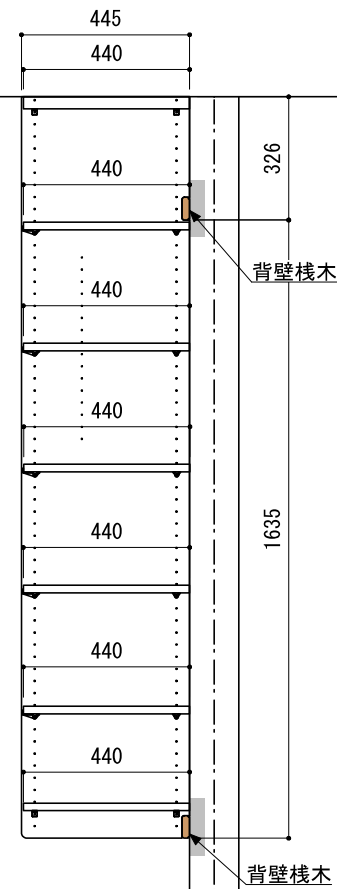
A-A' 断面
