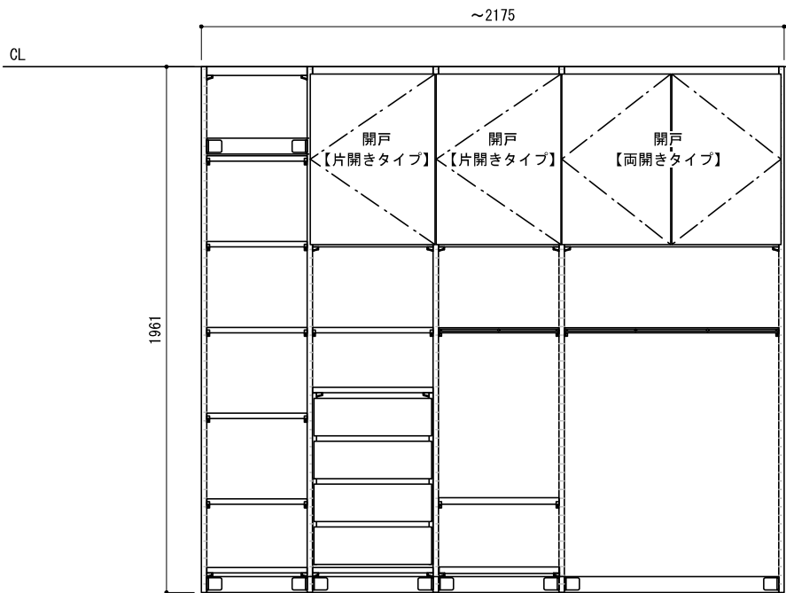
正面図（外観）
