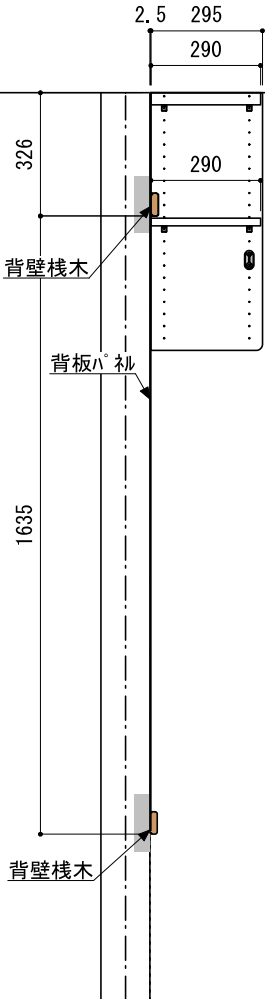
B-B' 断面
