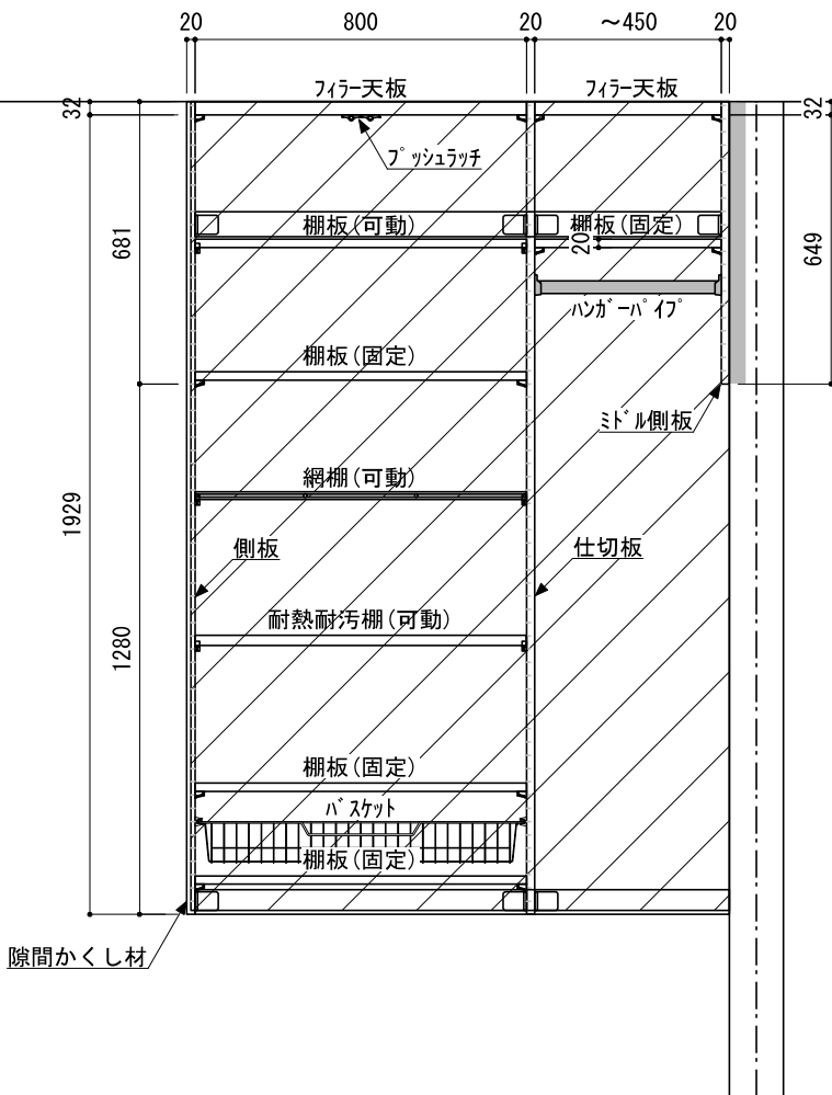
正面図（扉内部）
