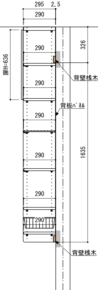
A-A' 断面
