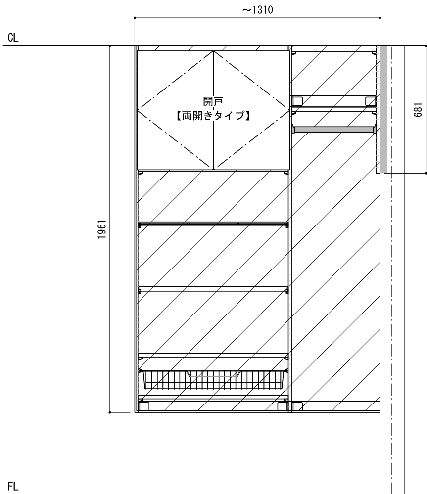
正面図（外観）
