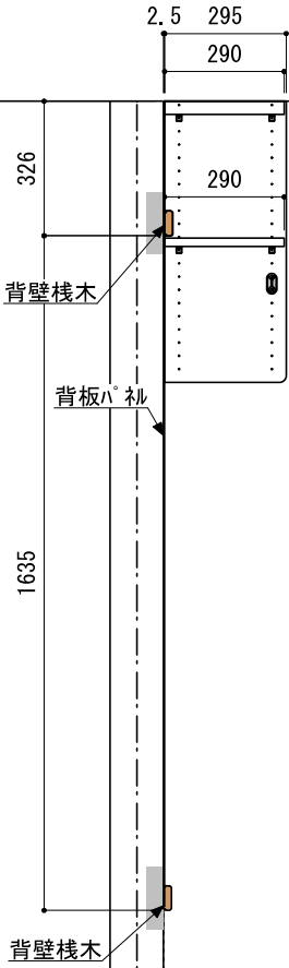
B-B' 断面
