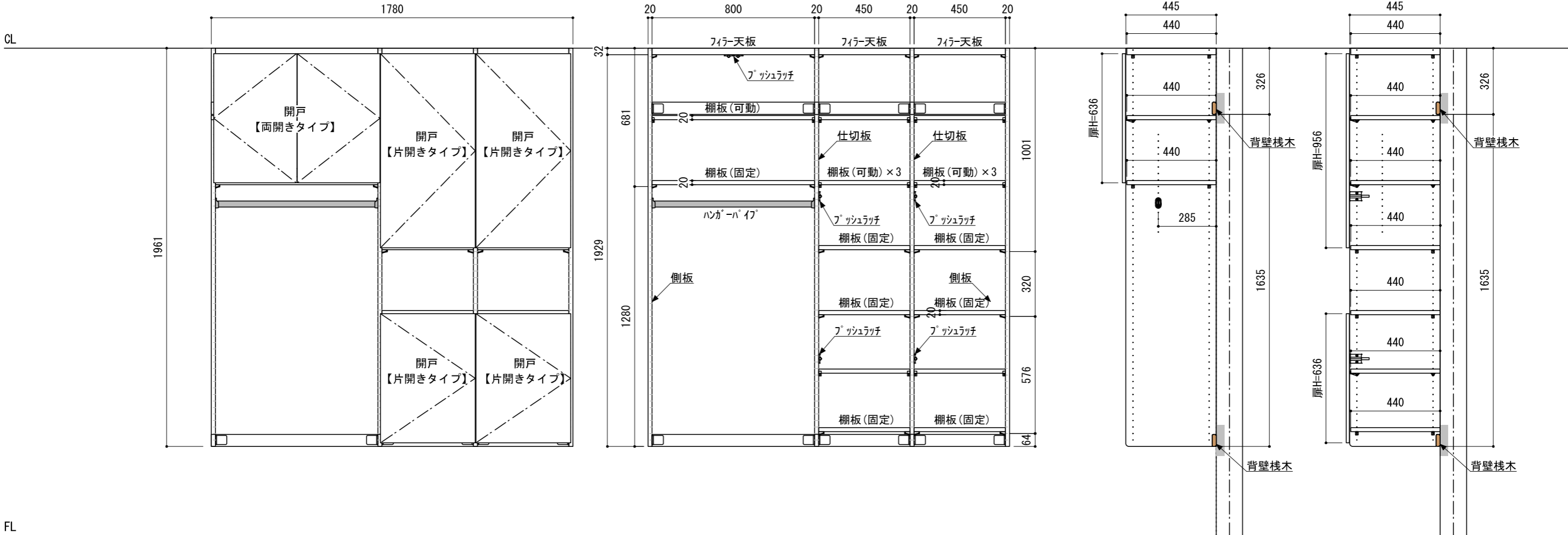
正面図（外観）
