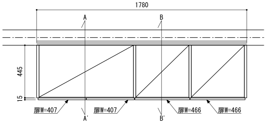
正面図（外観）
