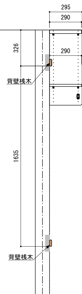
B-B' 断面
