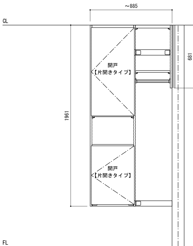
正面図（外観）
