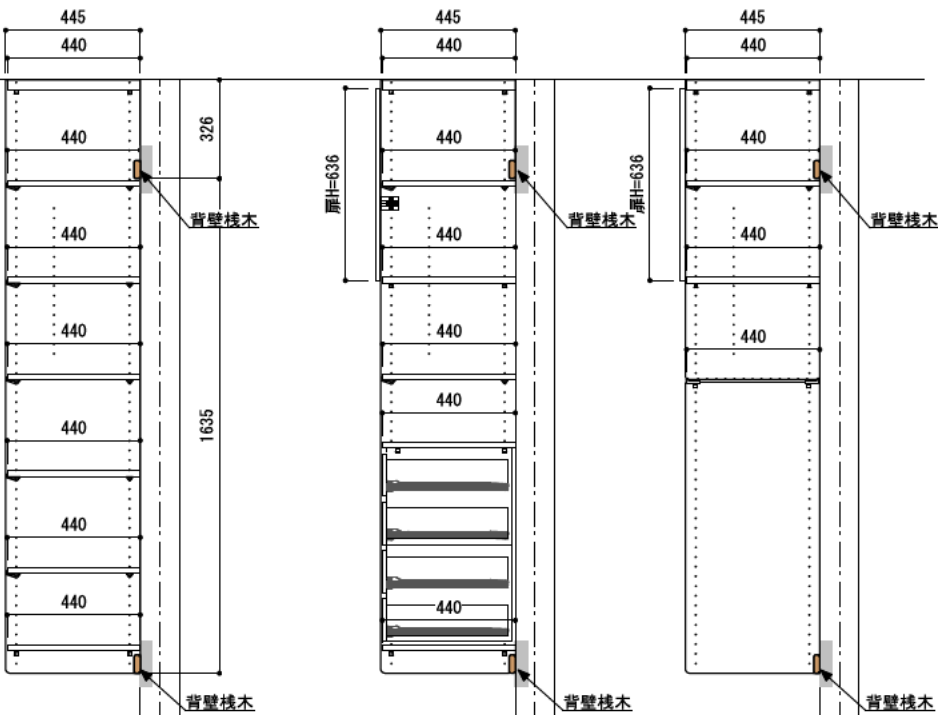
A-A' 断面
