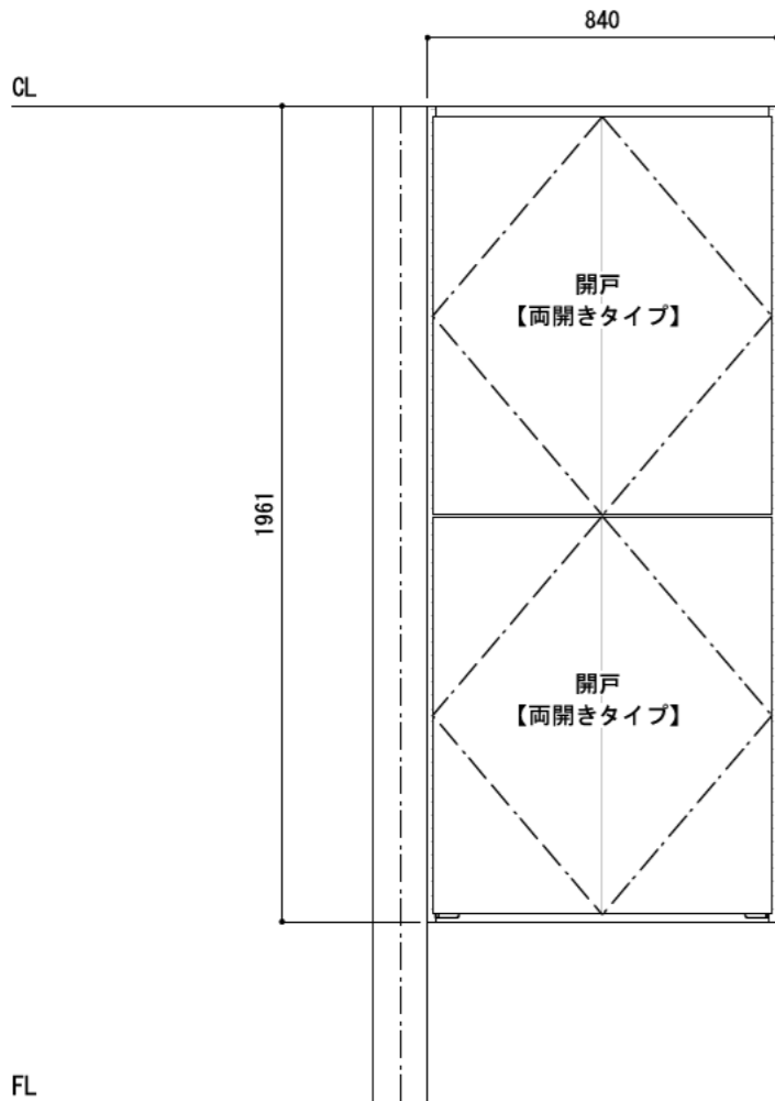
正面図 (外観)
