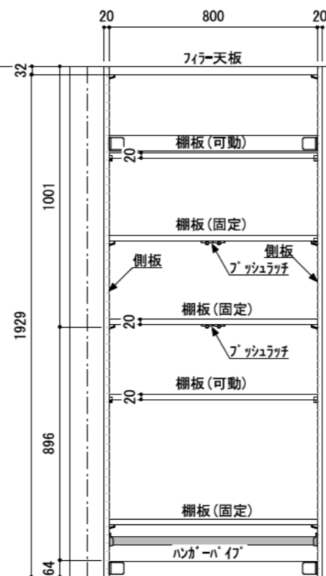
正面図 (扉内部)
