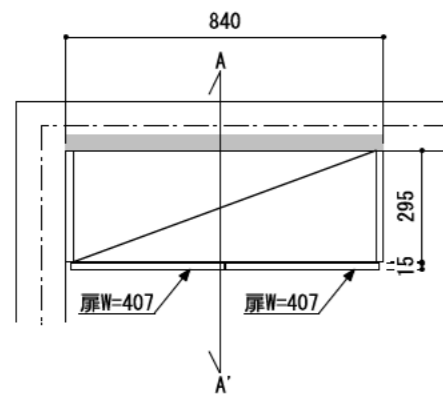
正面図 (外観)
