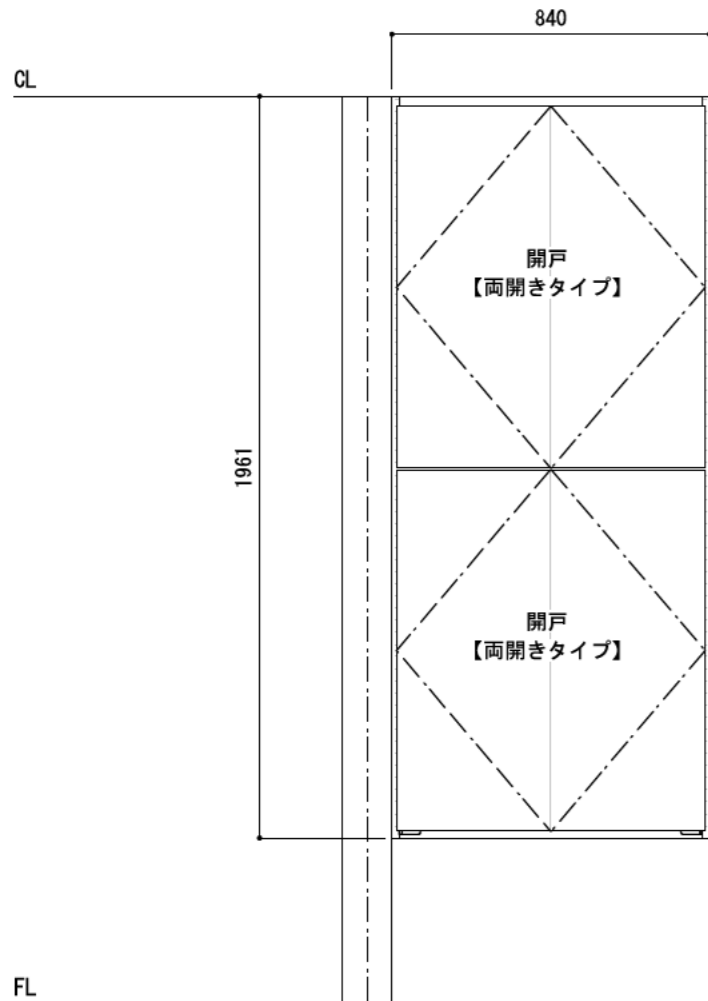
正面図（外観）
