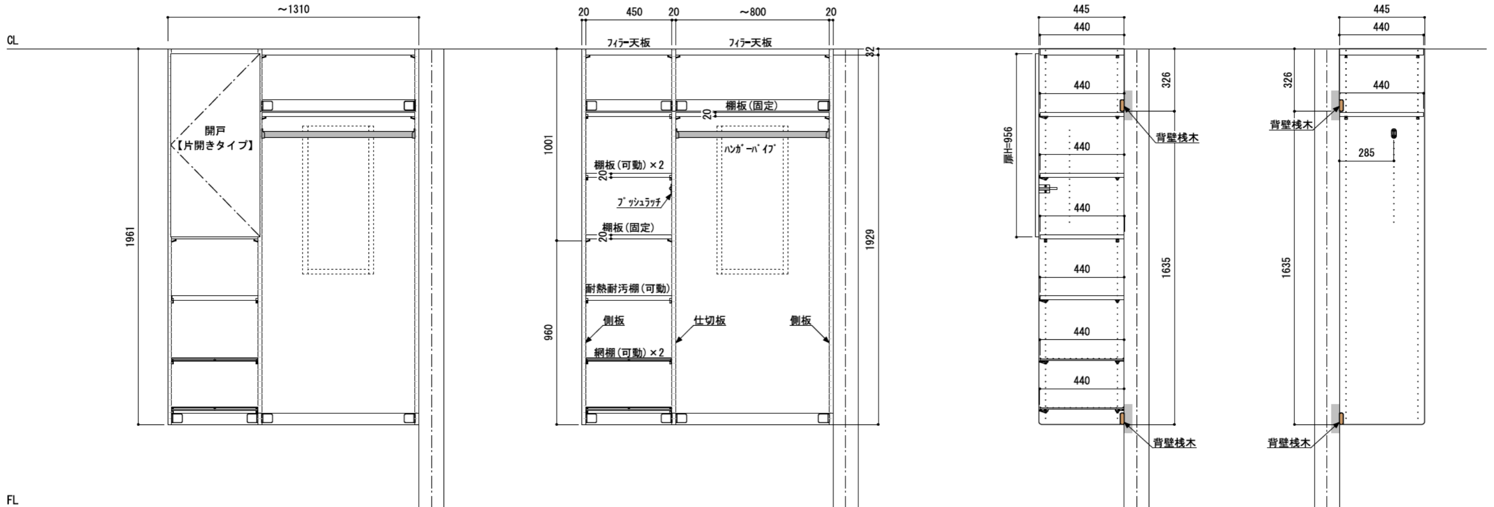
正面図（外観）
