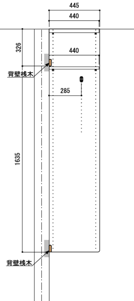
B-B' 断面
