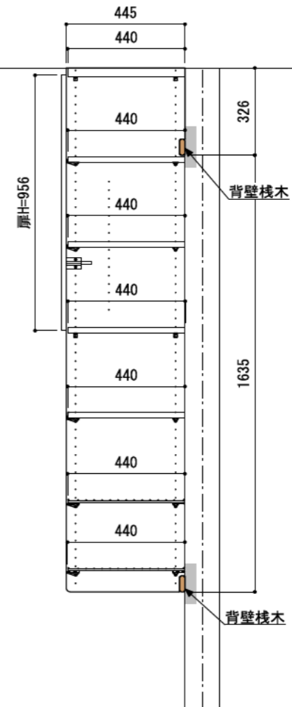
A-A' 断面
