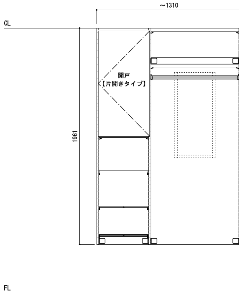
正面図（外観）
