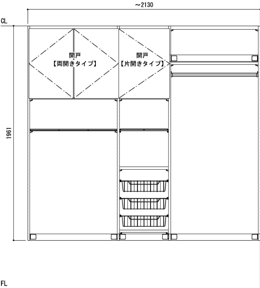
正面図（外観）
