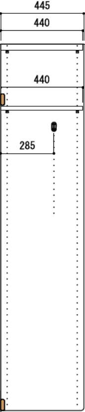
C-C' 断面
