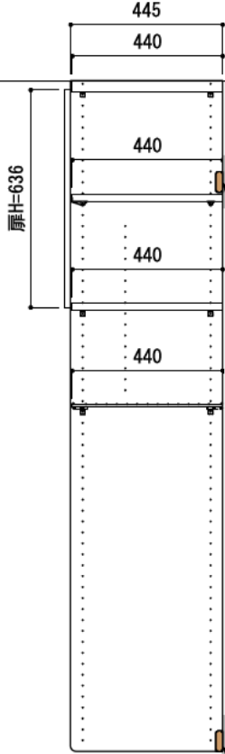
A-A' 断面
