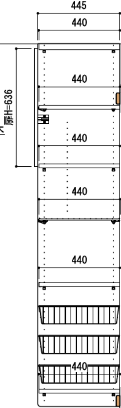
B-B' 断面
