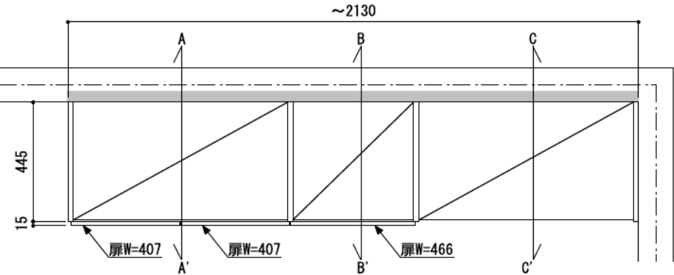
正面図（外観）
