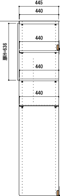
A-A' 断面
