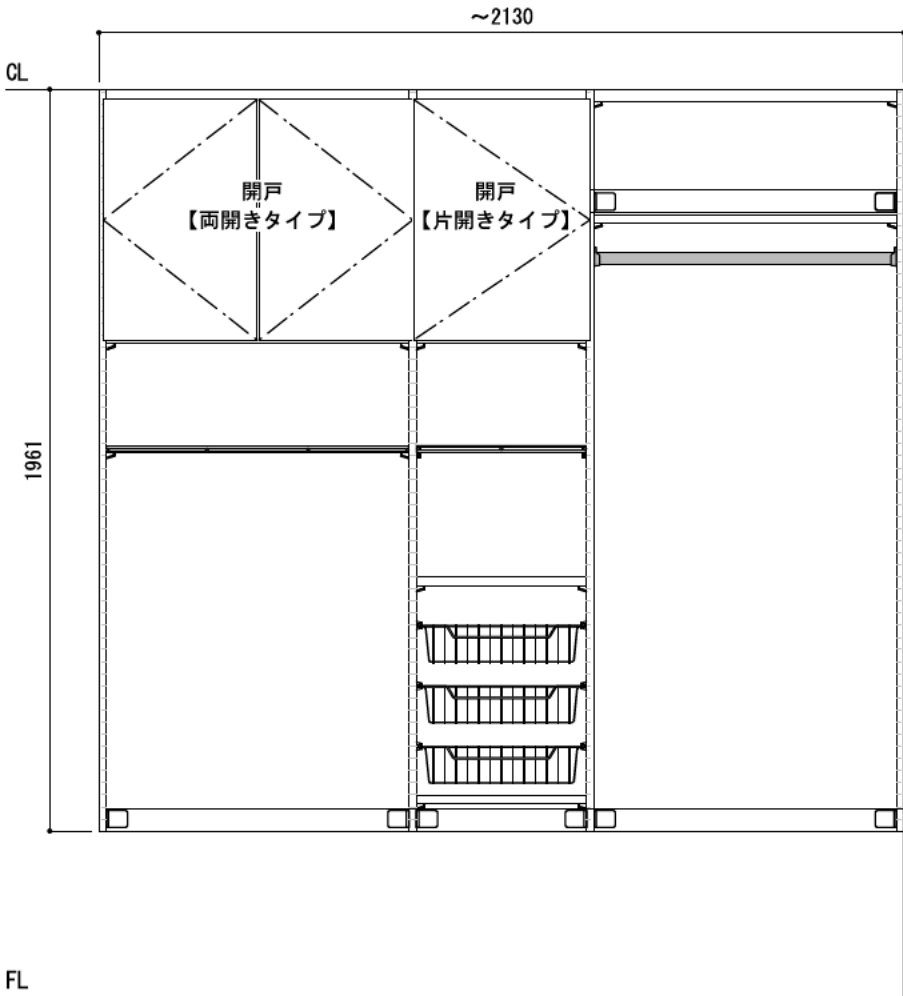
正面図（外観）
