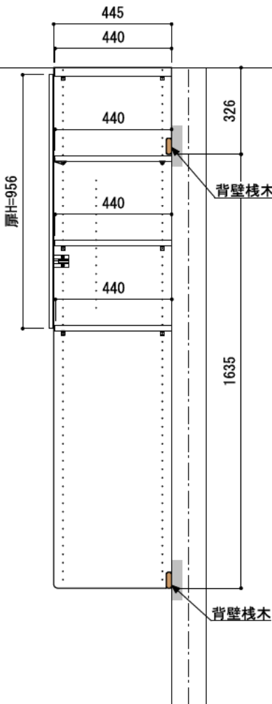
A-A' 断面
