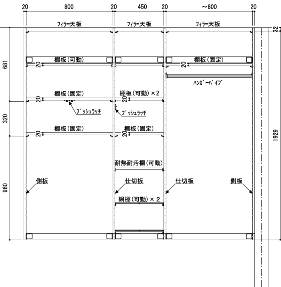
正面図（扉内部）
