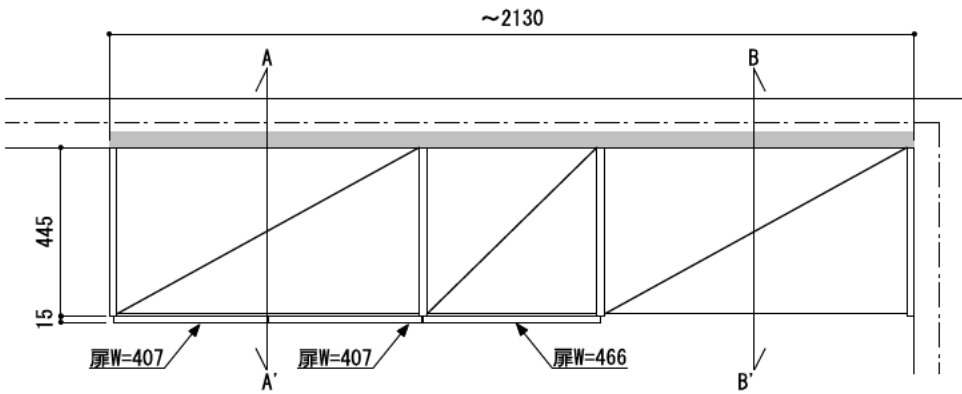
正面図（外観）
