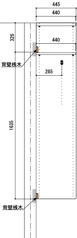
B-B' 断面
