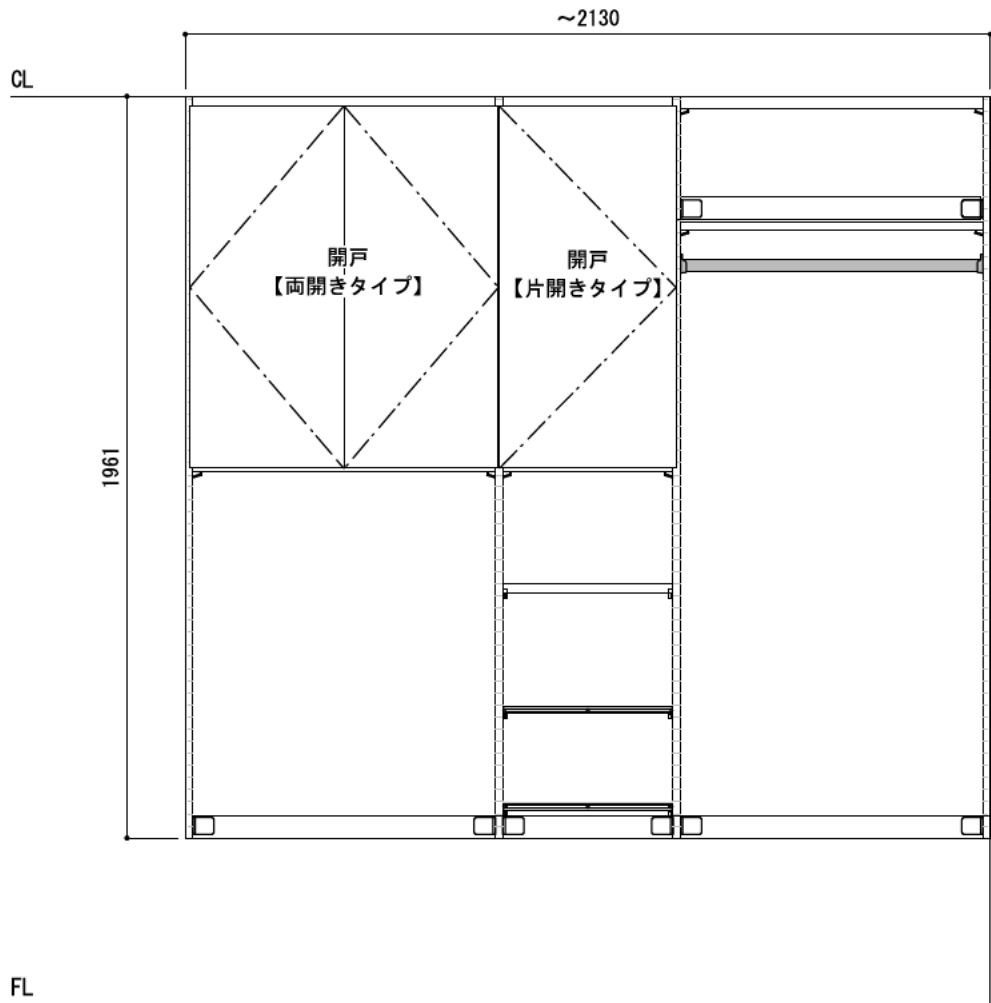
正面図（外観）
