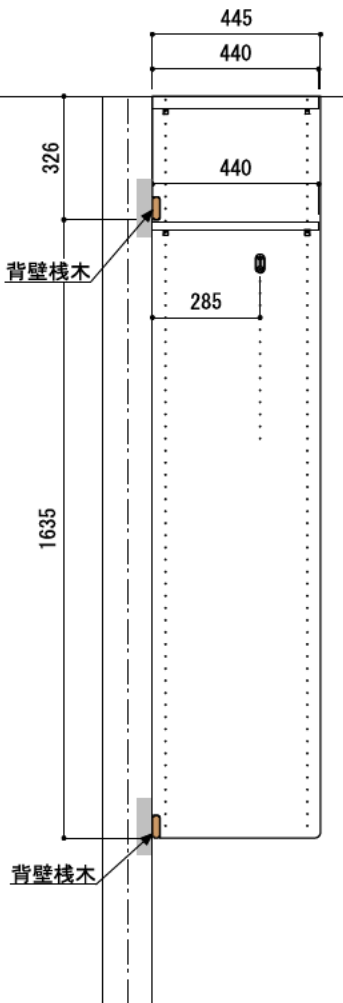
B-B' 断面
