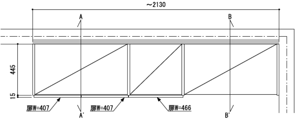
正面図（外観）
