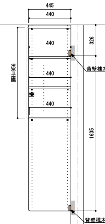
A-A' 断面
