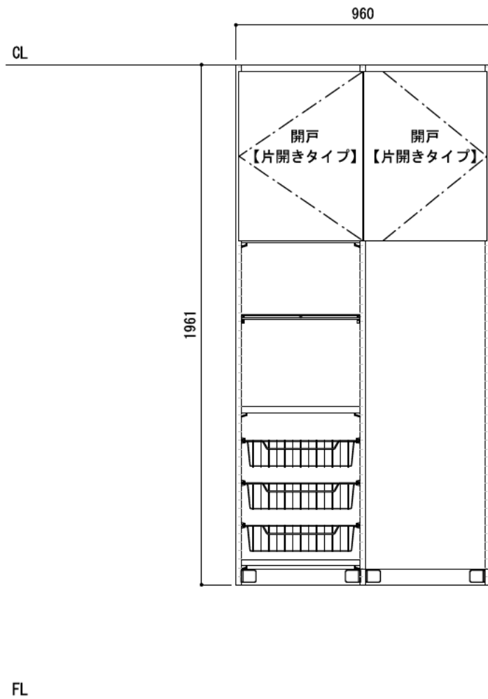
正面図（外観）
