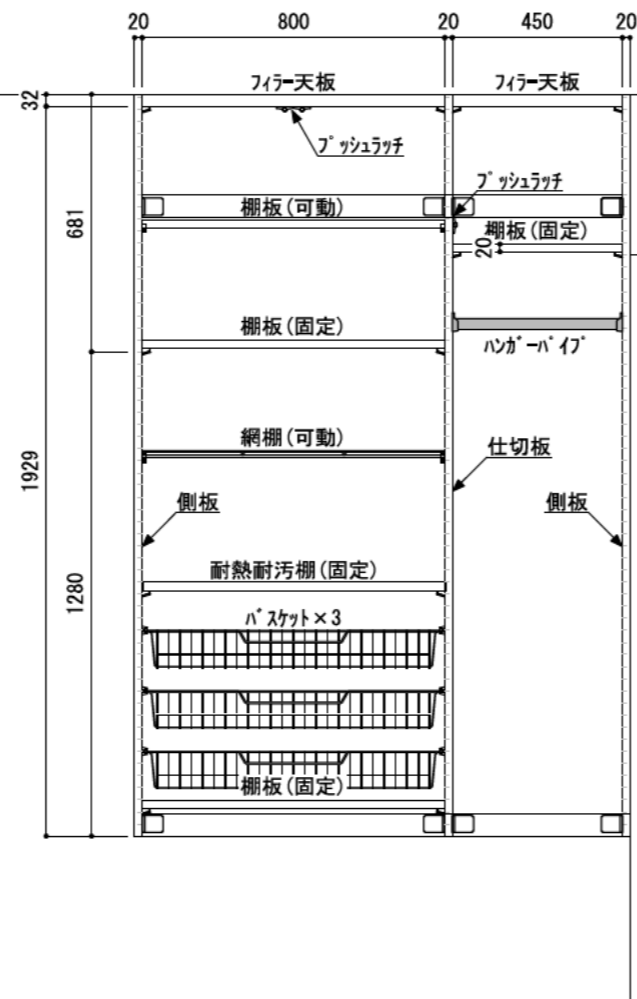
正面図（扉内部）
