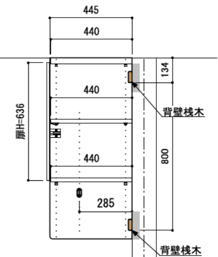
B-B' 断面
