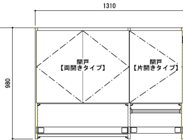
正面図（外観）
