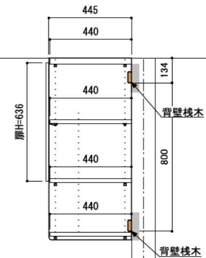
A-A' 断面
