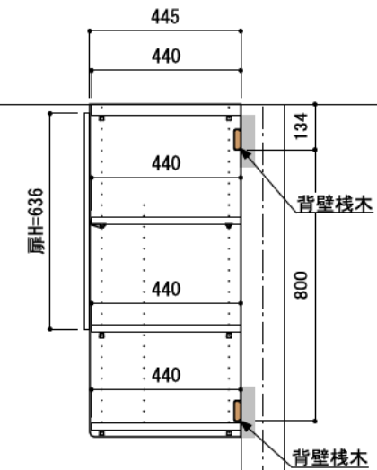
A-A' 断面
