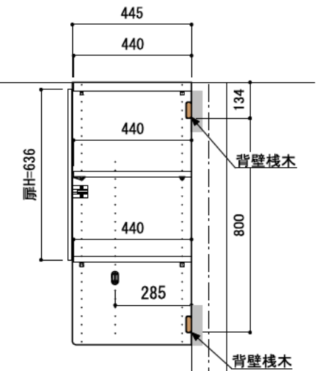
B-B' 断面
