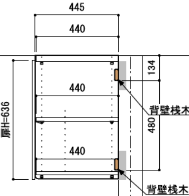
A-A' 断面
