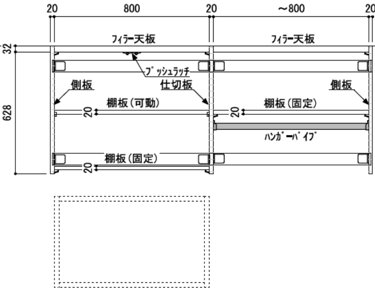
正面図（扉内部）
