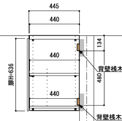
A-A' 断面
