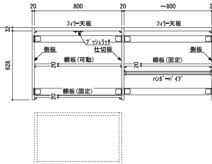
正面図（扉内部）
