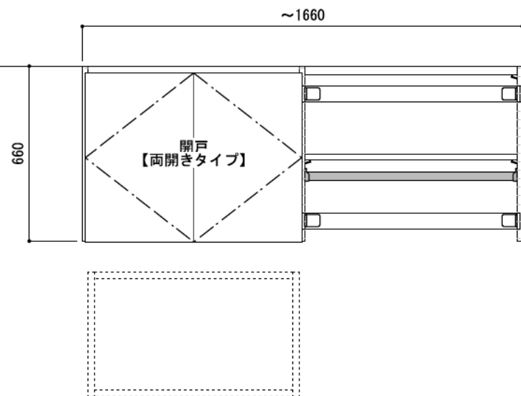
正面図（外観）
