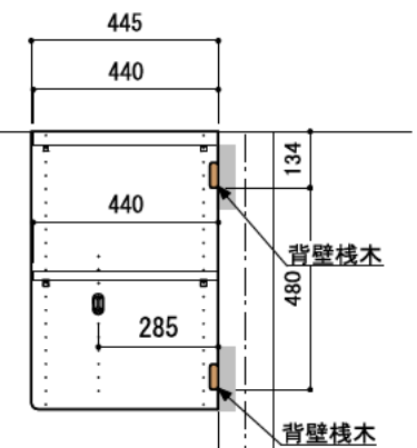
B-B' 断面
