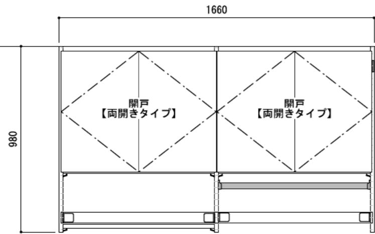
正面図（外観）
