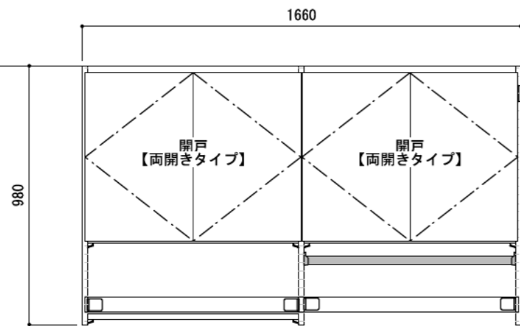
正面図（外観）
