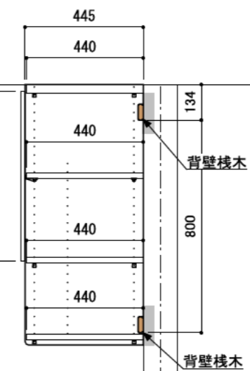
A-A' 断面
