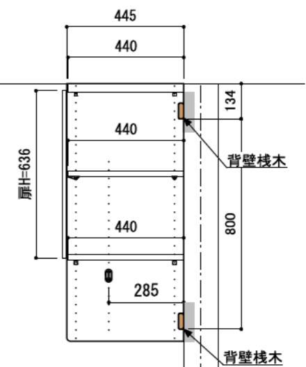
B-B' 断面
