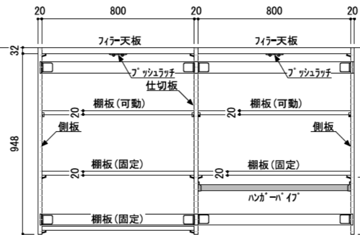
正面図（扉内部）
