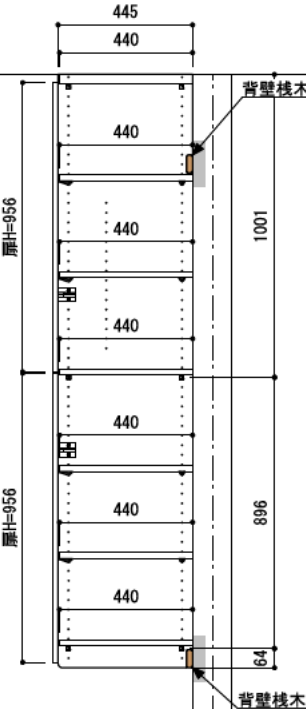
B-B' 断面
