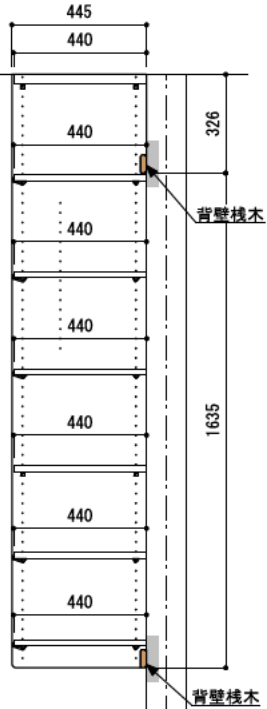
C-C' 断面
