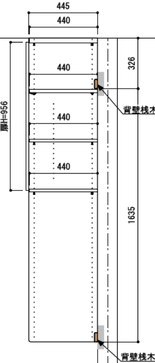
A-A' 断面
