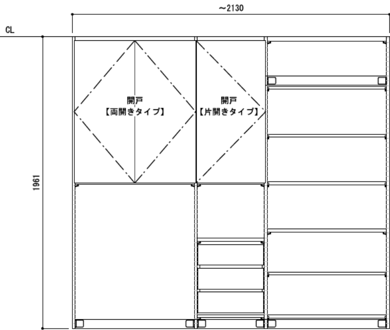
正面図（外観）
