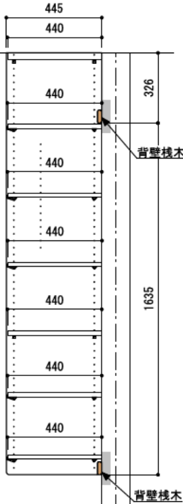
C-C' 断面
