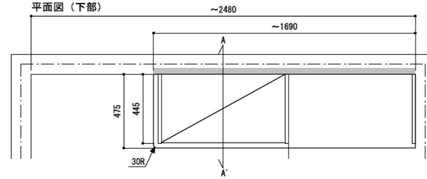
平面図（下部）
