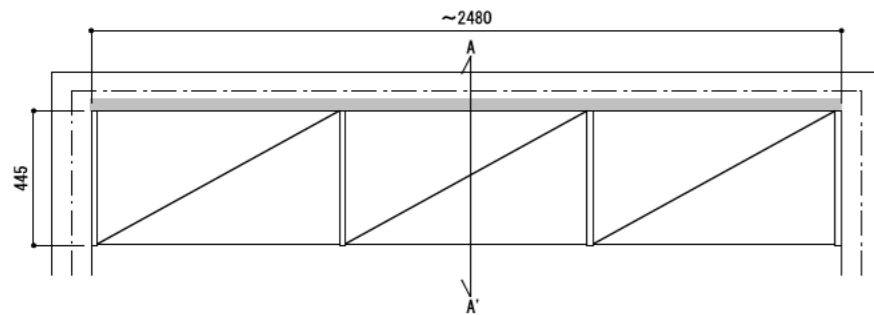
平面図（上部）
