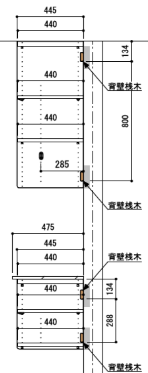
A-A' 断面
