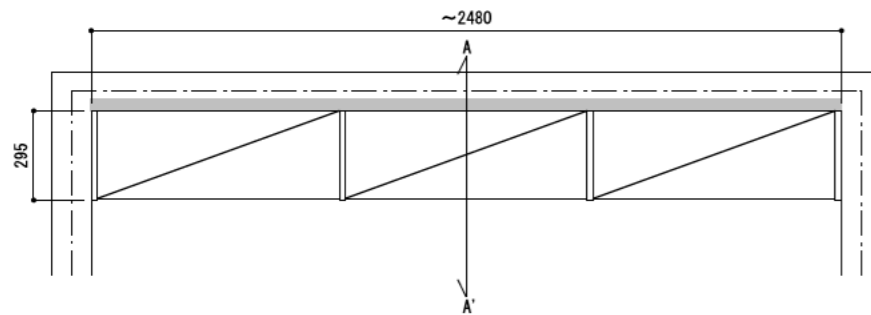
平面図（上部）
