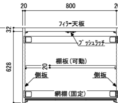
正面図（扉内部）
