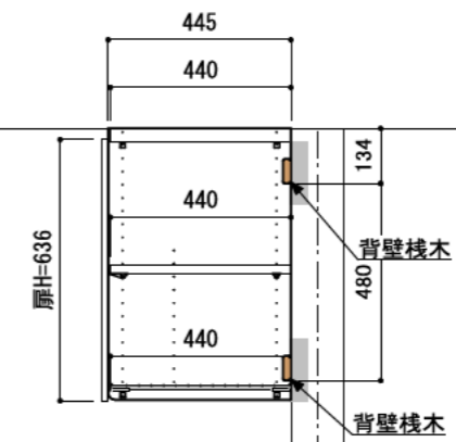
A-A' 断面
