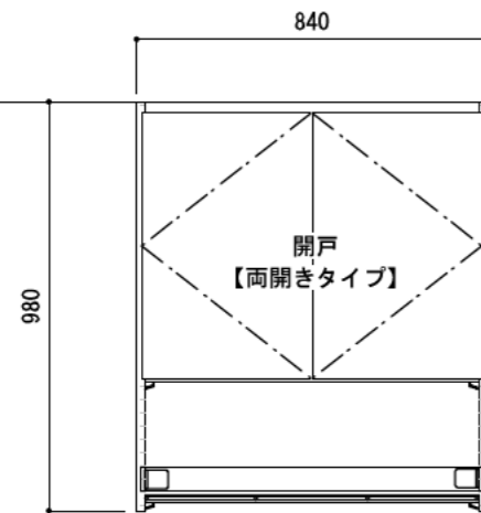
正面図（外観）
