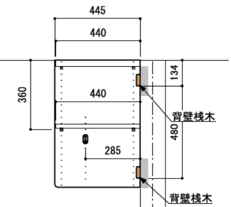
B-B' 断面
