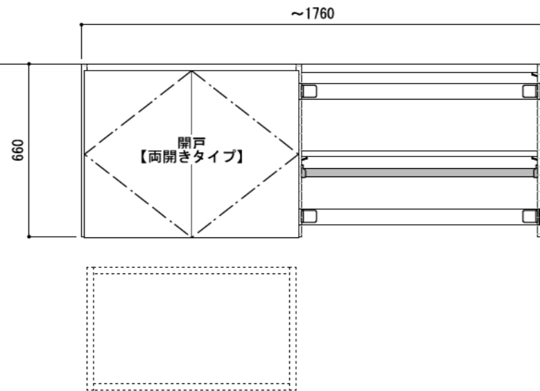
正面図（外観）
