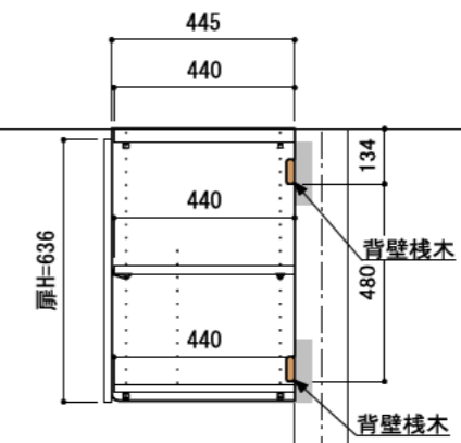
A-A' 断面
