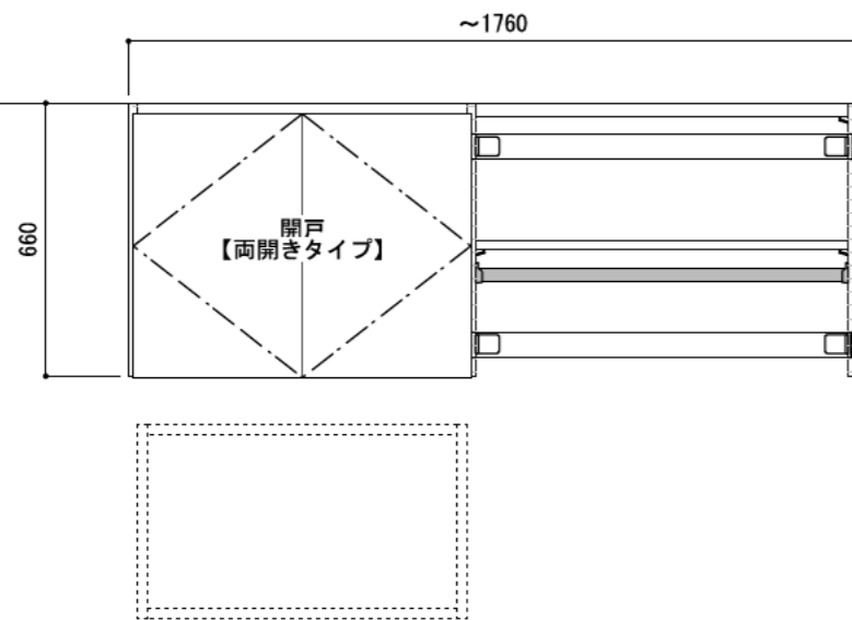
正面図（外観）
