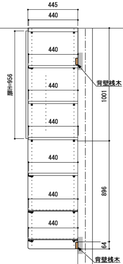
A-A' 断面
