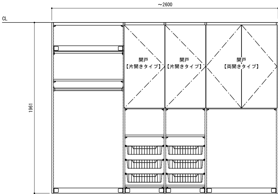
正面図（外観）
