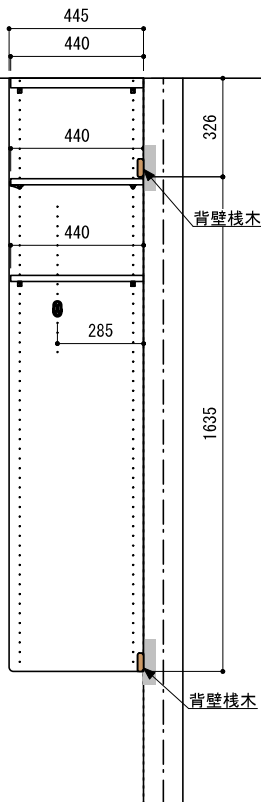
A-A' 断面
