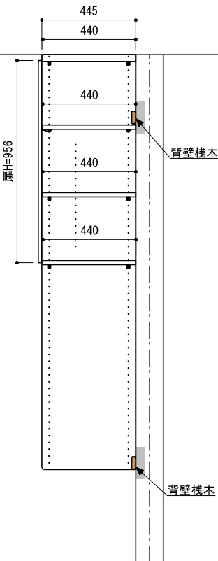
C-C' 断面
