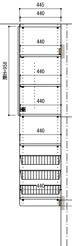
B-B' 断面
