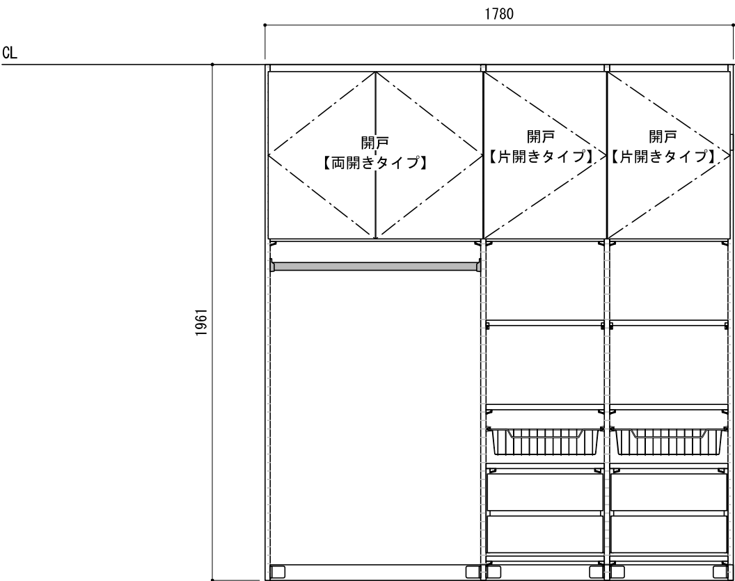
正面図（外観）
