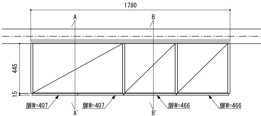
正面図（外観）
