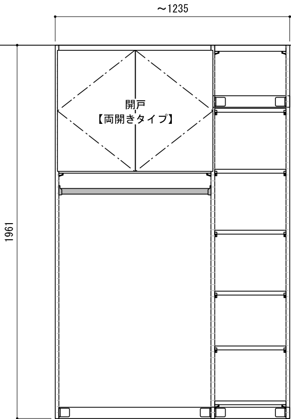
正面図（外観）
