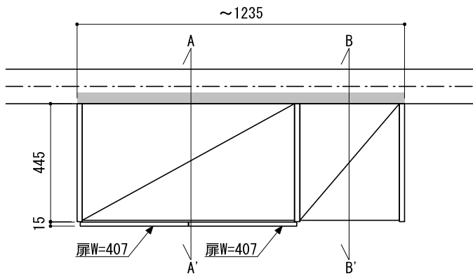
正面図（外観）
