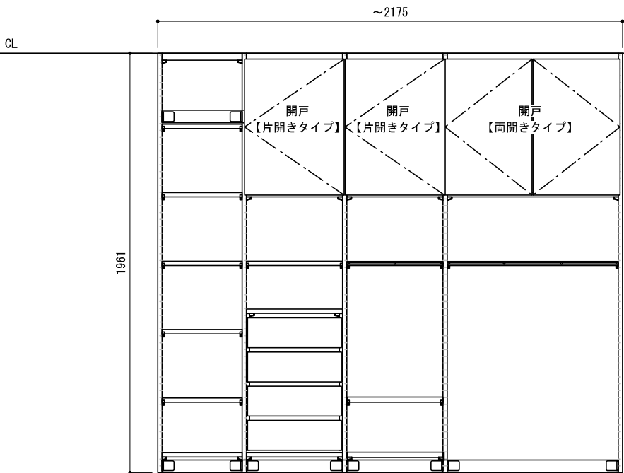
正面図（外観）
