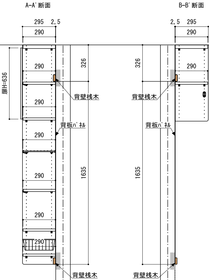
A-A' 断面
