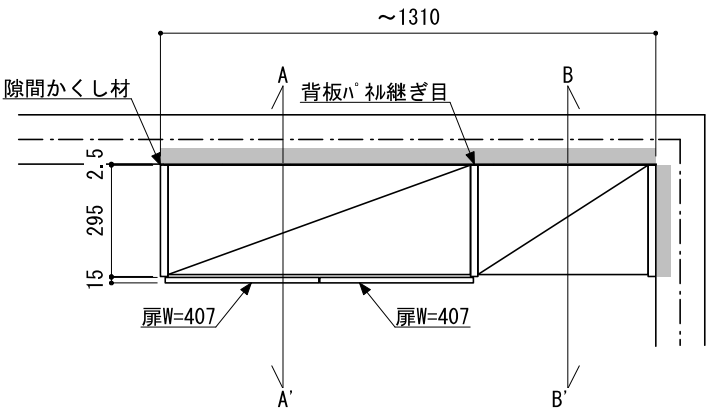
正面図（外観）
