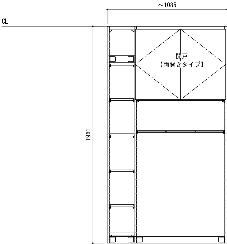
正面図（外観）
