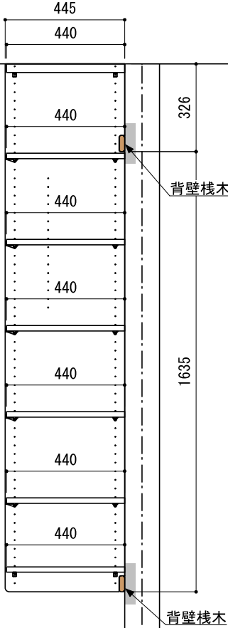
A-A' 断面
