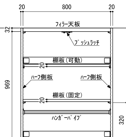
正面図（扉内部）
