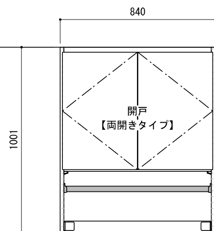
正面図（外観）
