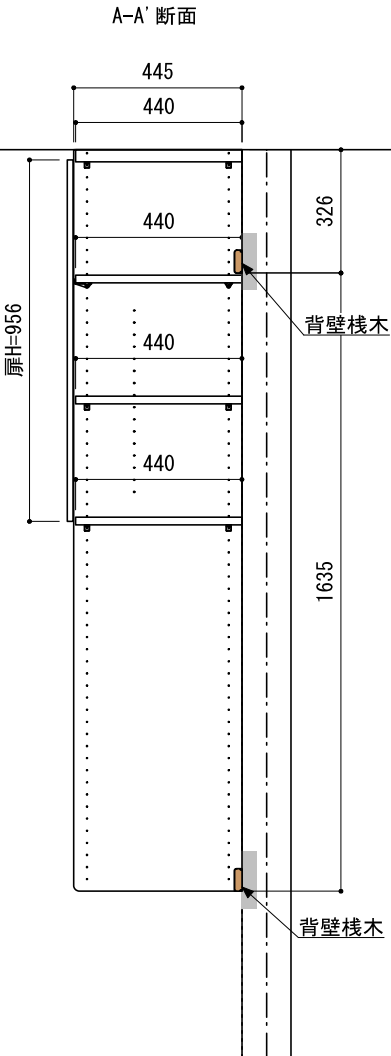
A-A' 断面
