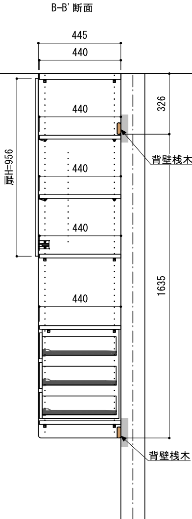
B-B' 断面
