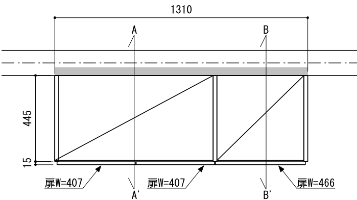
正面図（外観）
