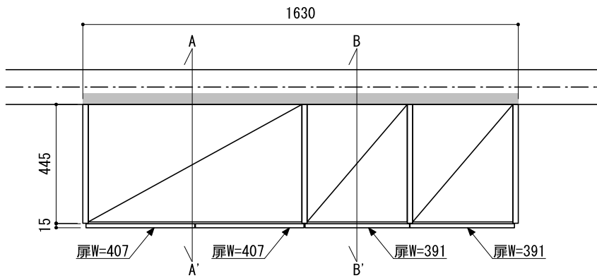
正面図（外観）
