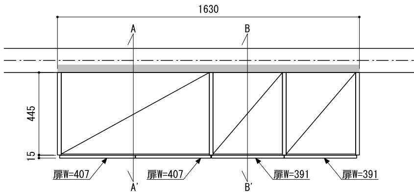
正面図（外観）
