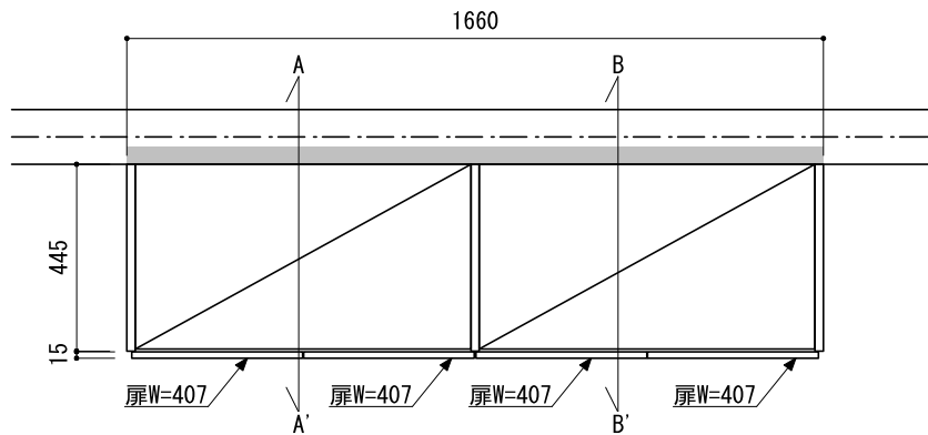
正面図（外観）
