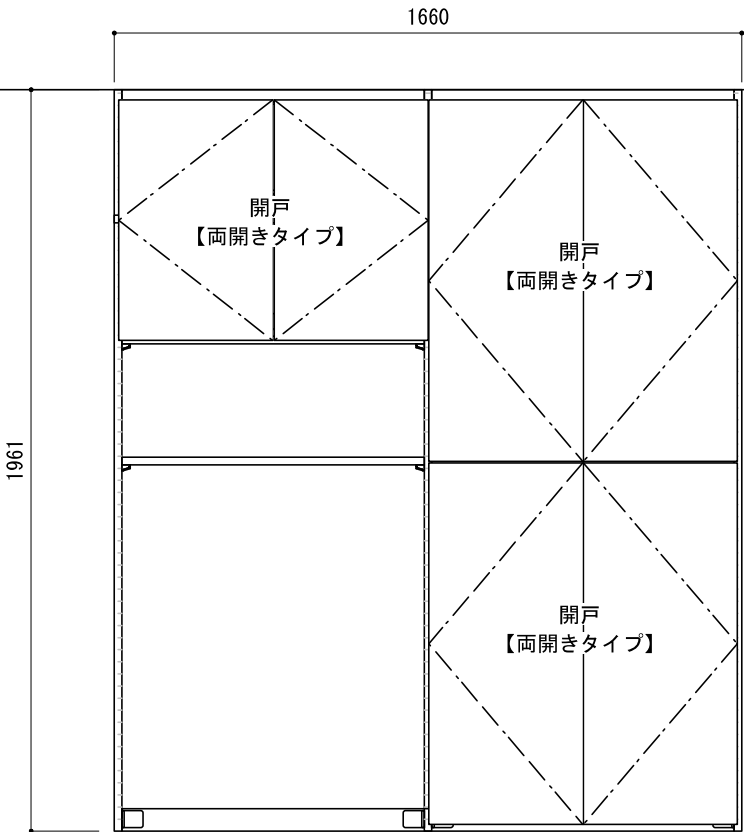
正面図（外観）
