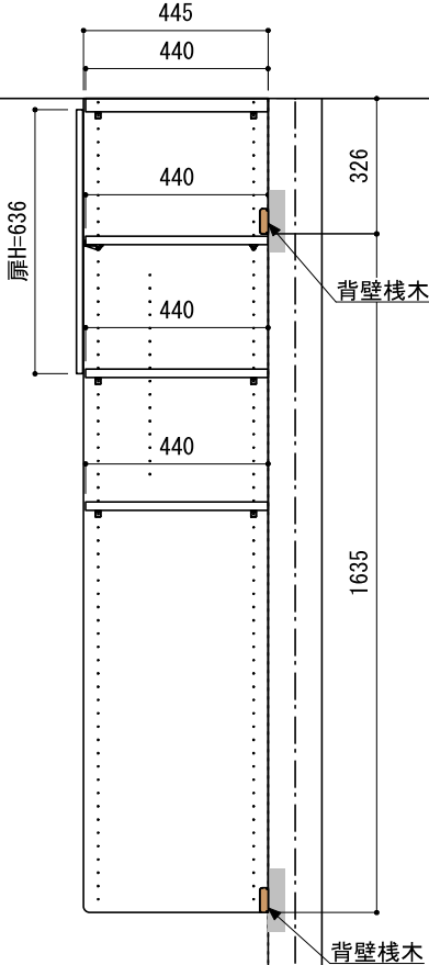
A-A' 断面
