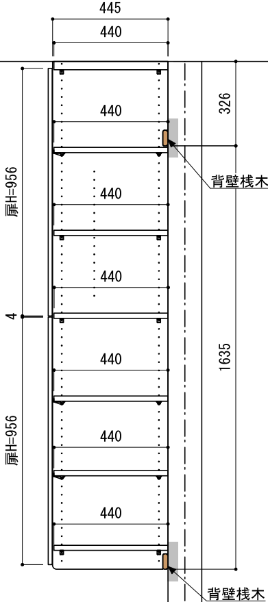
B-B' 断面
