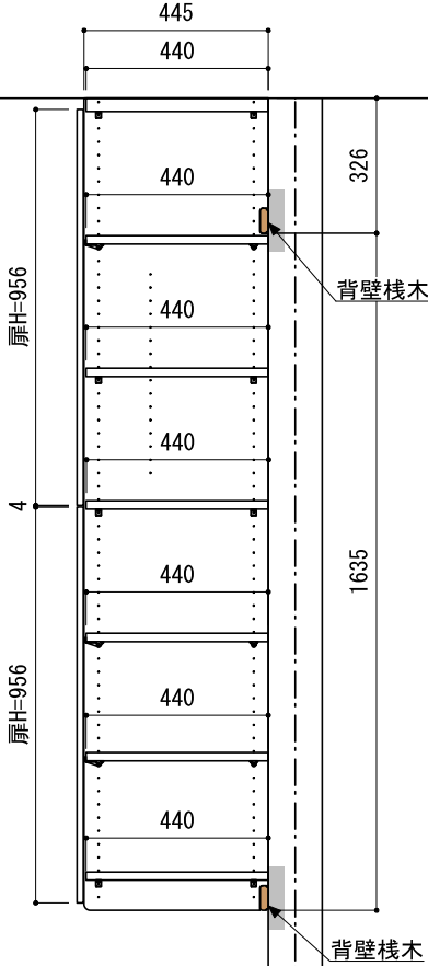
B-B' 断面
